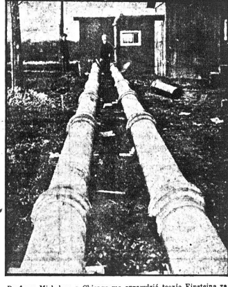
Professor Michelson z Chicago ma sprawdzić teorię Einsteina za pomocą aparatu powyżej sfotografowanego
